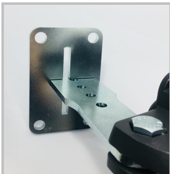
Sposób montażu blachy na wąskim słupku
